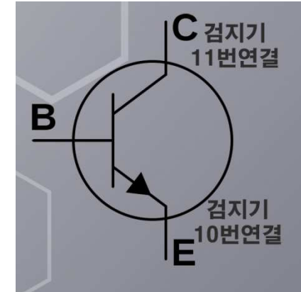
별첨: NPN형 감지기 연결법
